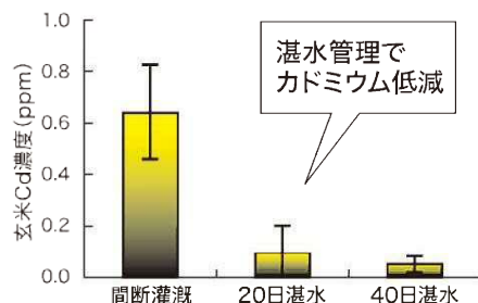
図2 水管理と玄米カドミウム濃度
