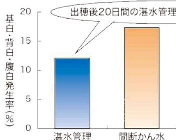
図1 出穂後の水管理と玄米品質
